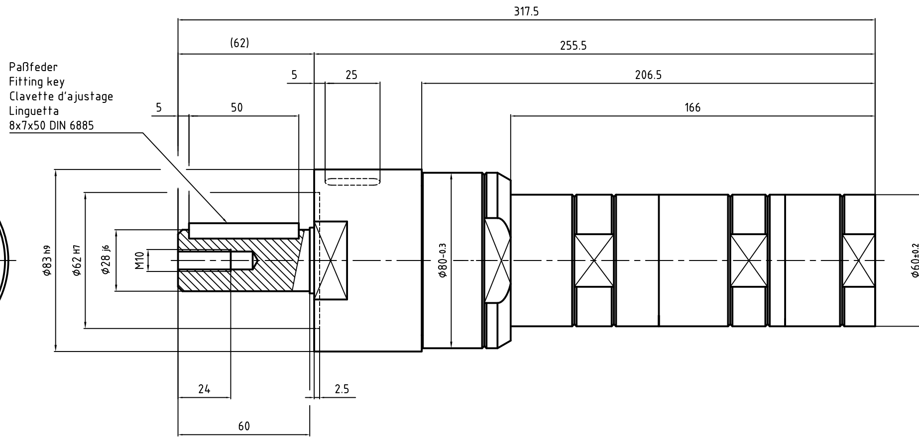
Motor MRD 120-65 60002215
